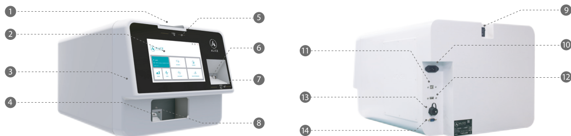
1. Entrada de moedas, 2. Ecrã / touchscreen, 3. Porta da máquina, 4. Saída de moedas, 5. Led indicativo de validador de moedas ativo, 6. Entrada e saída de notas, 7. Led indicativo de validador de notas ativo, 8. Fechadura oculta para abertura da porta, 9. Botão para ligação da máquina [ON/OFF], 10. Conetor cabo de alimentação, 11. Conetor cabo OTG, 12. Conetor cabo USB, 13. Conetor Ethernet, 14. Conetor de serviço RS232.
